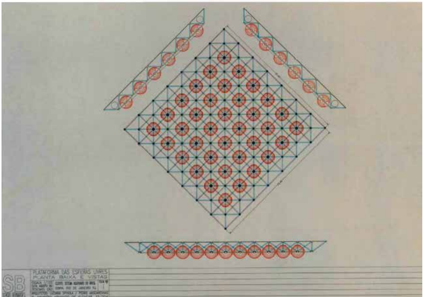
Plataforma de transporte marítimo sobre esferas livres
